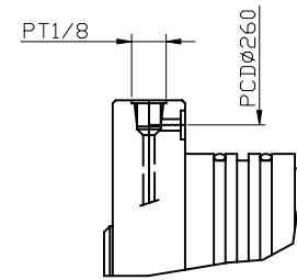
前端氣幕
